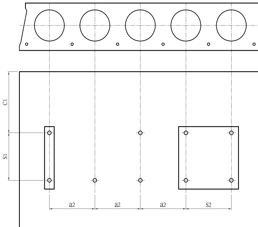
Figura B3. Parámetros de instalación para anclajes en losas alveolares de hormigón.
