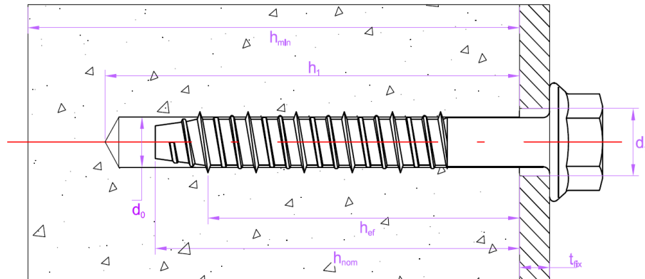
Figura A1. Condiciones de instalación en hormigón para anclajes SSW, SSR, SSP, SSK, SSH, SSX, SST, SSN y SSC.
