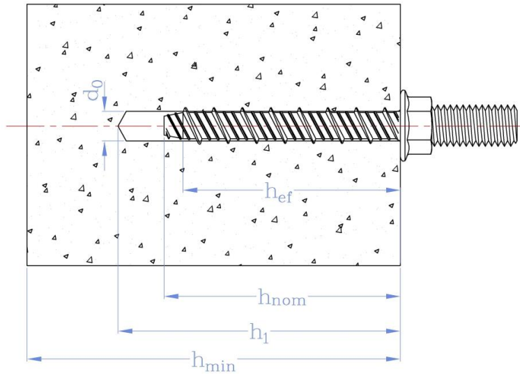
Figura A3. Condiciones de instalación para anclajes SSD, SSI, SSF, SSO, SSU, SSG, SSQ, SSV and SSG2 en bloques de hormigón
