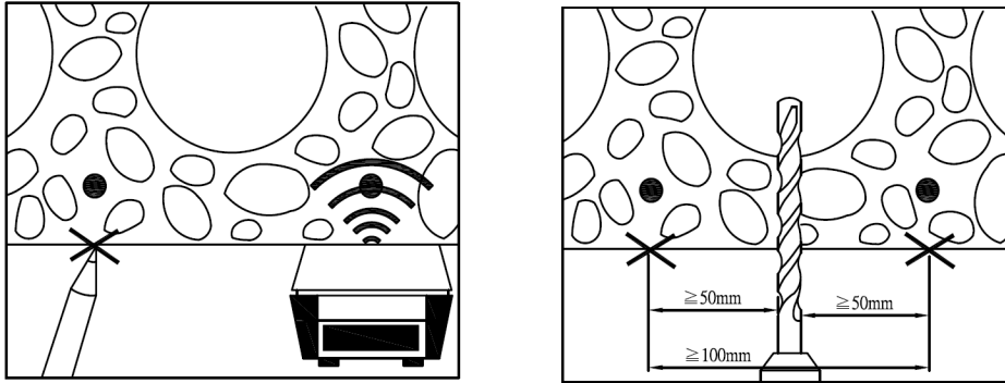
Figura B4. Proceso de instalación en losa alveolares
