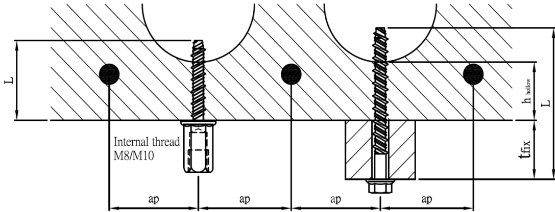
Figura A4. Condiciones de instalación para anclajes en losas alveolares de hormigón
