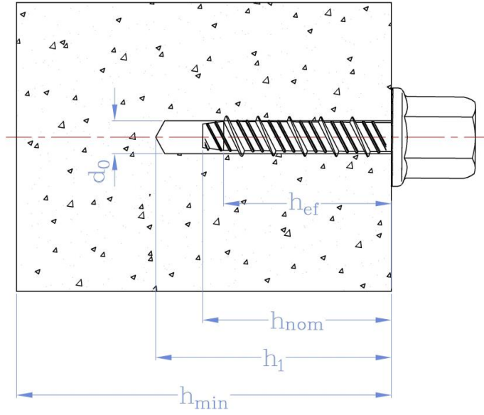
Figura A2. Condiciones de instalación para anclajes SSD, SSI, SSF, SSO, SSU, SSG, SSQ, SSV and SSG2 en bloques de hormigón
