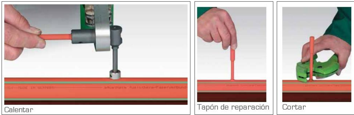
Figura 4. Reparación con varilla
