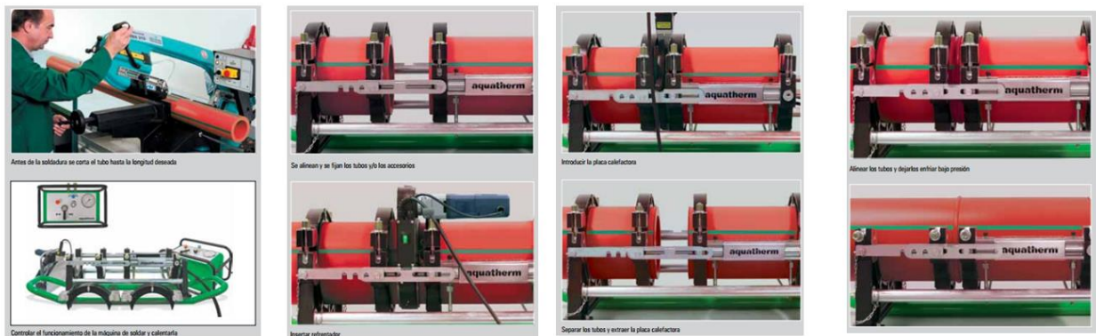
Figura 2.1. Soldadura con termofusión: soldadura a tope. Proceso
