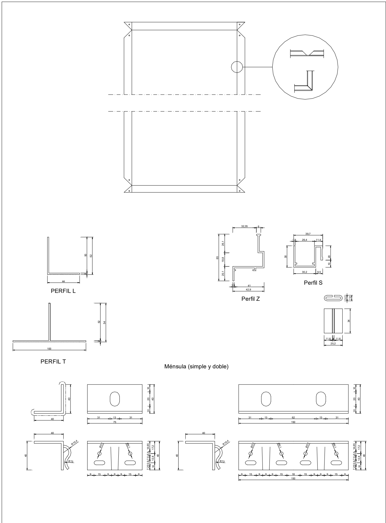
Figura 2. Detalles de formación de bandeja (arriba) y de componente de subestructura (abajo)
