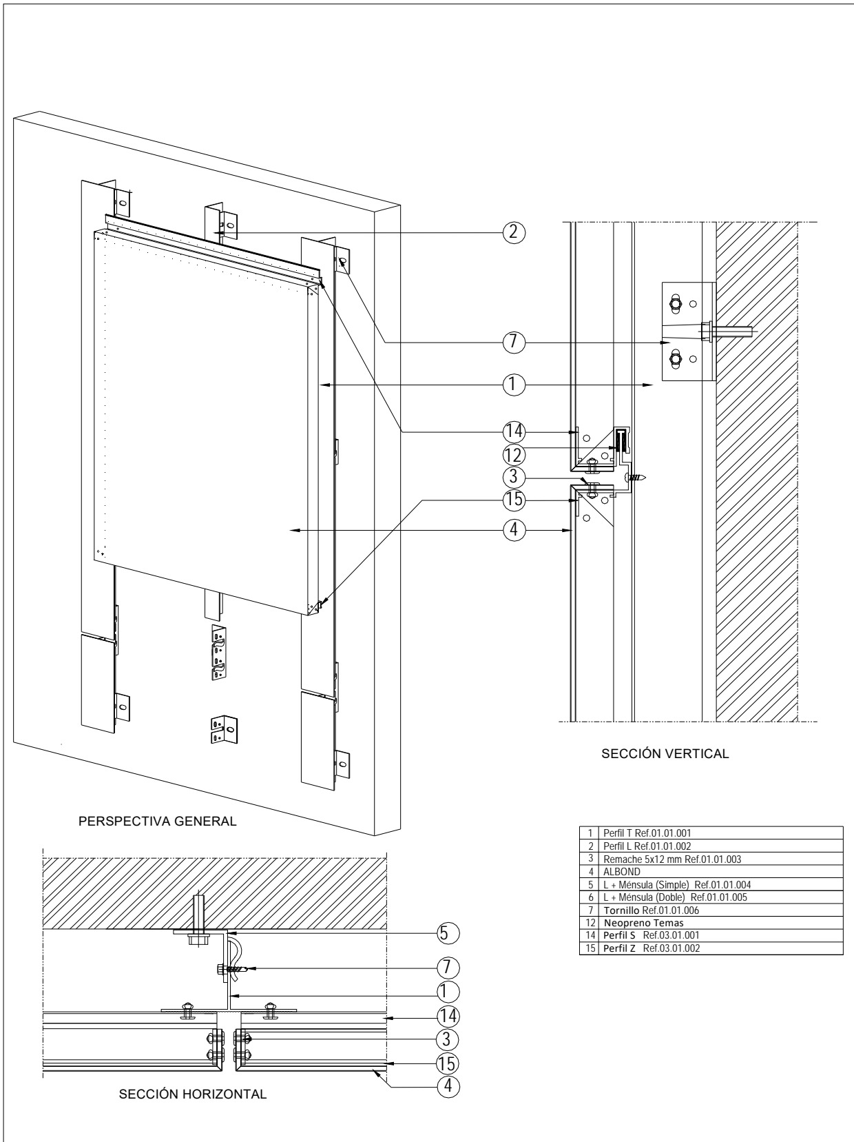
Figura 1: Esquemas del kit ALBOND SZ
