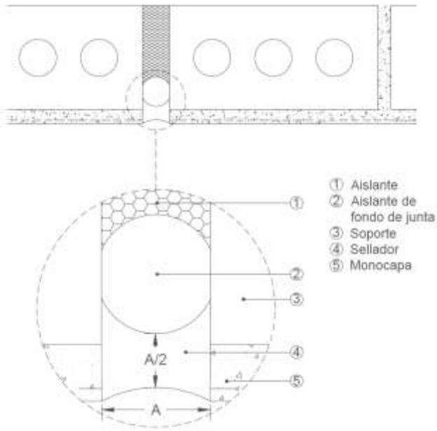
Fig. 1. Solución de la junta estructural
