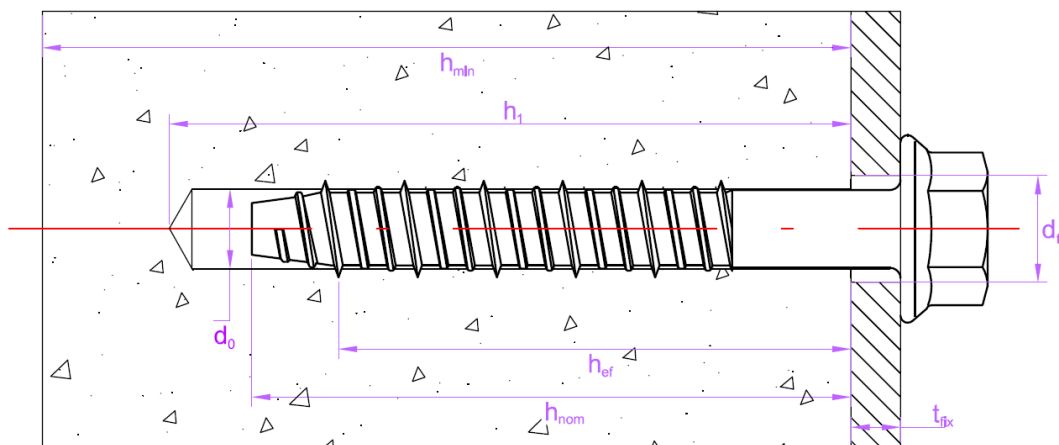
Figura A1. Esquema de instalación para anclajes CS-W y CS-C.
