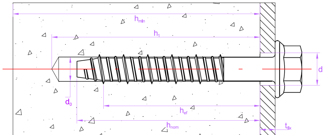
Figura B1. Esquema de instalación para anclajes CS-W y CS-C.
