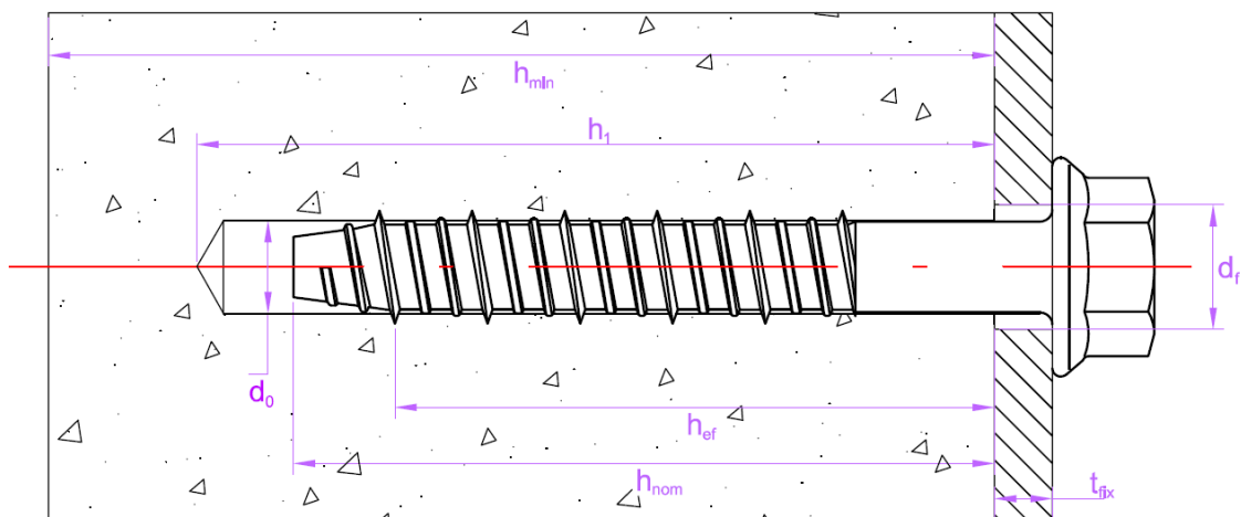
Figura B1. Esquema de instalación para anclajes 07070 (W), 07085 (R), 07080 (P), 07090 (K), 07071 (H), 07073 (X), 07082 (T) and 07083 (N).
