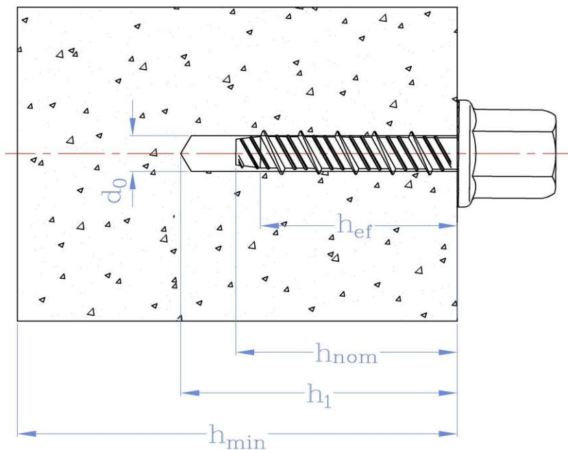
Figura A2. Esquema de instalación para anclajes 60010 (D), 63073 (I), 60020 (F), 60070 (O), 60033 (U), 63071 (G), 63070 (Q) and 63075 (V).
