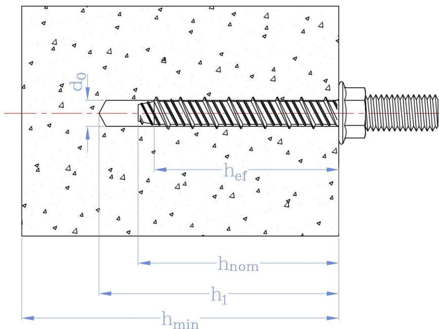
Figura A3. Esquema de instalación para anclajes 60010 (D), 63073 (I), 60020 (F), 60070 (O), 60033 (U), 63071 (G), 63070 (Q) and 63075 (V).
