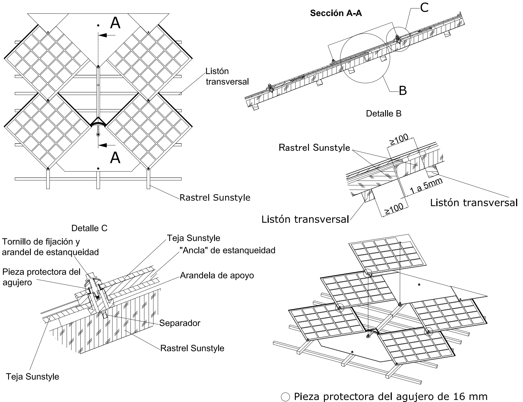
Figura 9 – Juntas entre tramos de rastreles Sunstyle y piezas protectoras de los agujeros de 16 mm de los módulos
