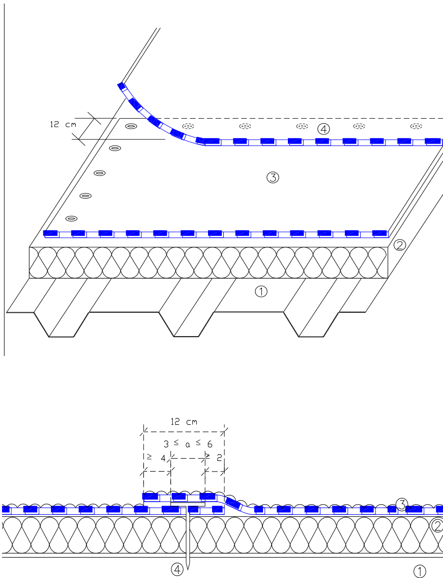
Fig. 1 Detalle del solape de las láminas.
